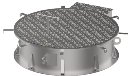
HUBER Schachtabdeckung SD7.R RC4.
