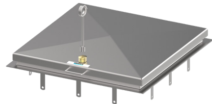
HUBER Schachtabdeckung SD3 RC3.
